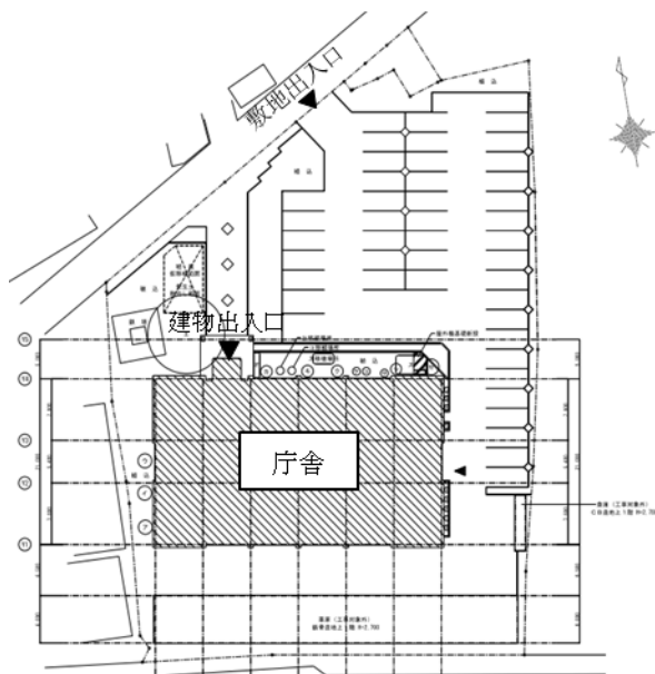
配置図
