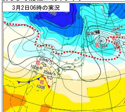
実況天気図
