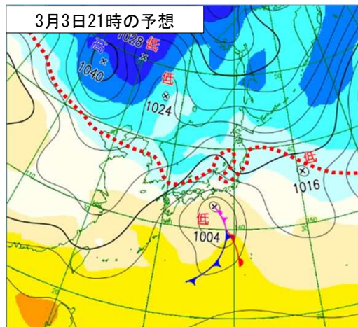
予想天気図
