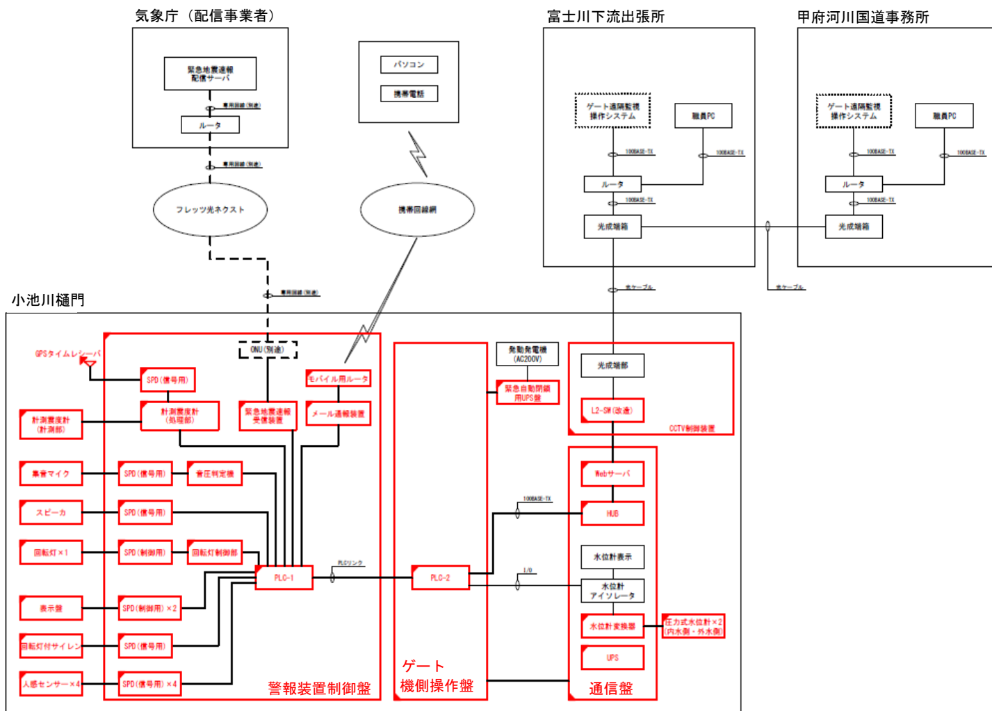
【システム構成図】
