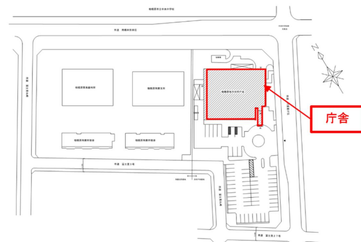
配置図
