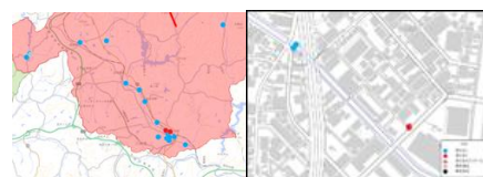
実証実験中の浸水センサ及び表示システム
