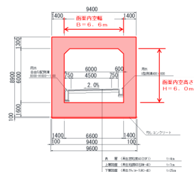
標準断面図
