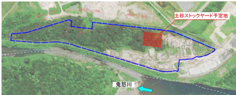
土砂ストックヤード整備 平面図（塩野室地区）
