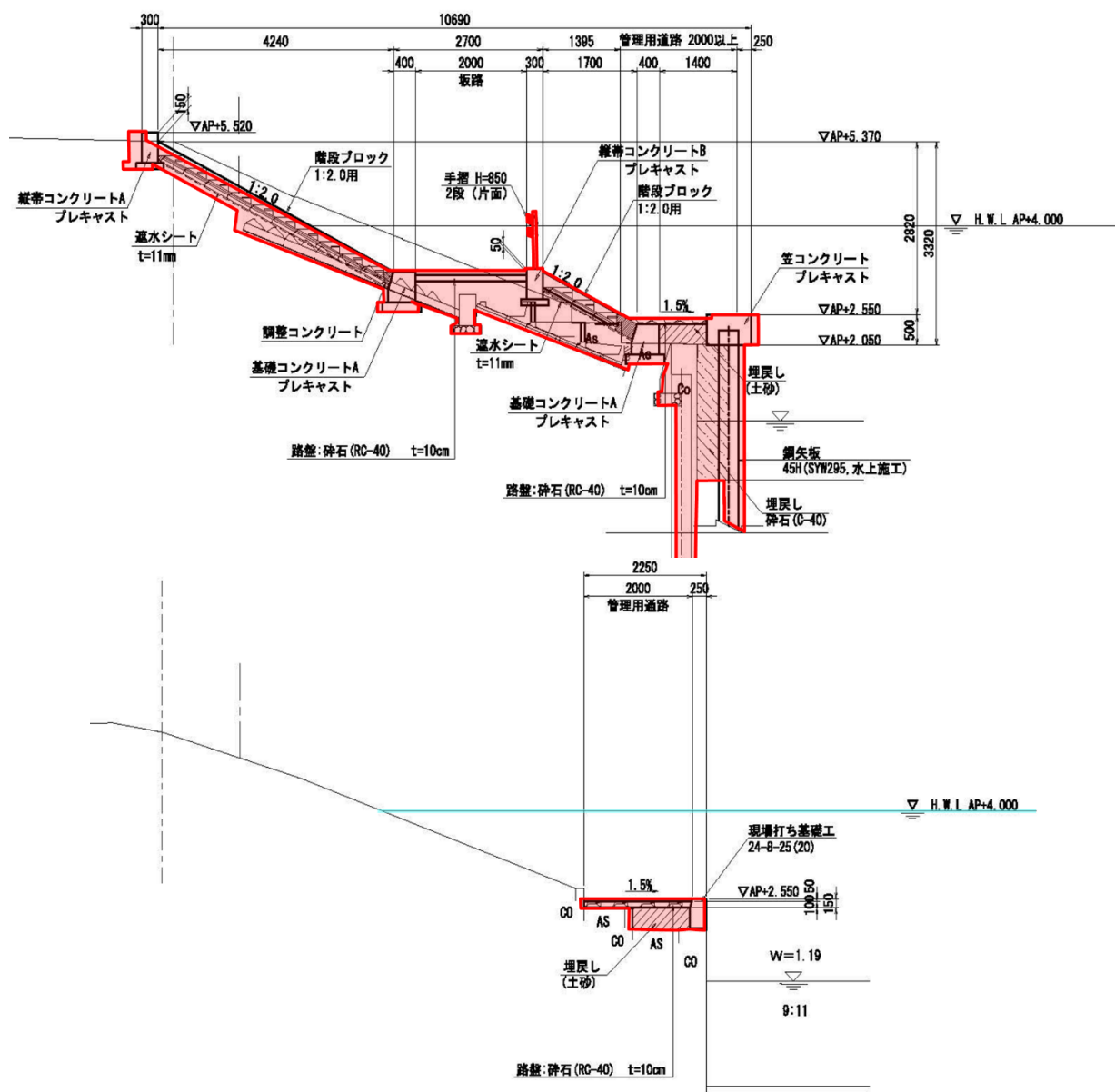
標準横断図
