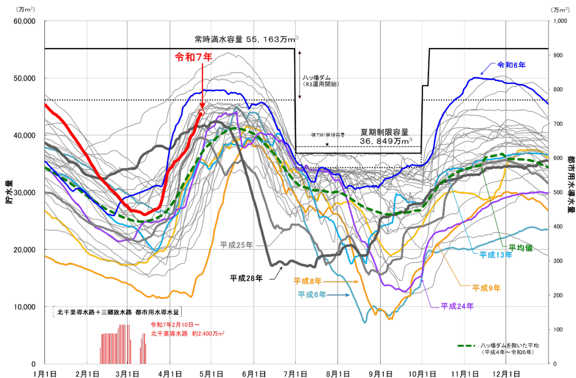
図-9 利根川上流 9 ダム貯水容量図 (令和 7 年 4 月 23 日 0 時現在)
