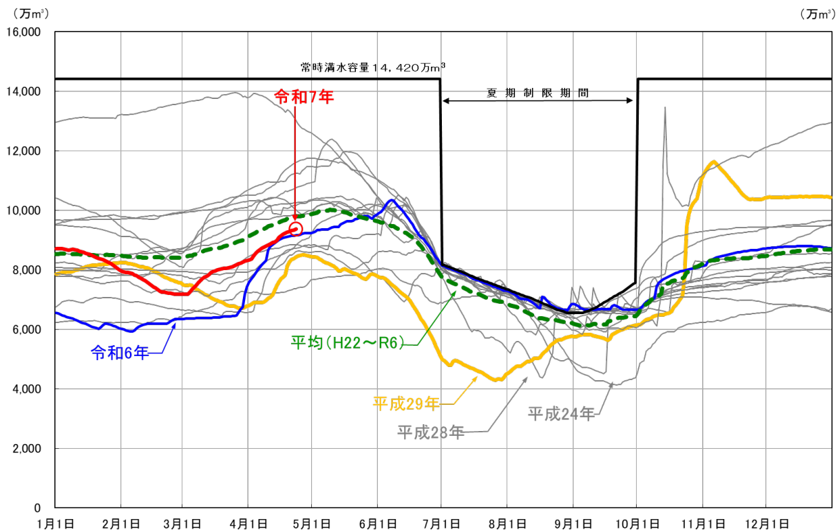
図-16 荒川4ダム貯水量図（令和7年4月23日0時現在）
