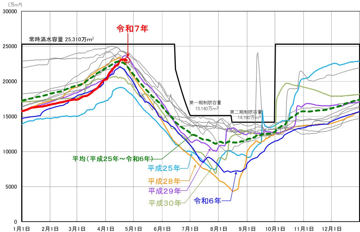
図-14 鬼怒川上流4ダム貯水容量図(令和7年4月23日0時現在)
