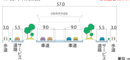
標準断面図
