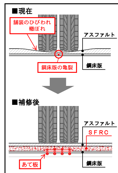
鋼床版の補修イメージ
