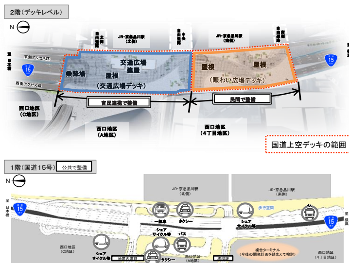
施設配置計画と官民の事業区分
