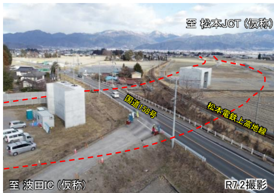
まつもと にいむら 松本市新村地区の工事状況
