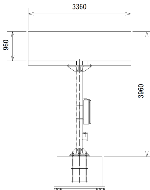
外観イメージ（河川情報板）
