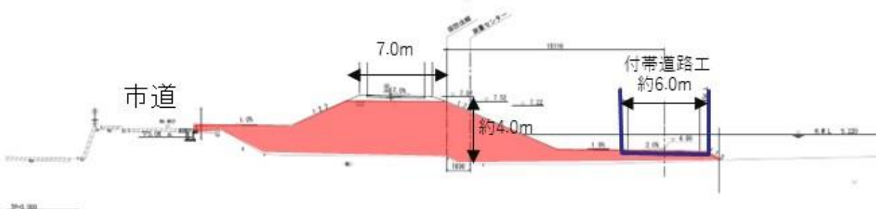
横断面図
