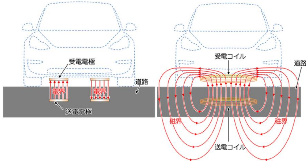
非接触給電におけるイメージ (左:電界結合方式 右:磁界結合方式)
