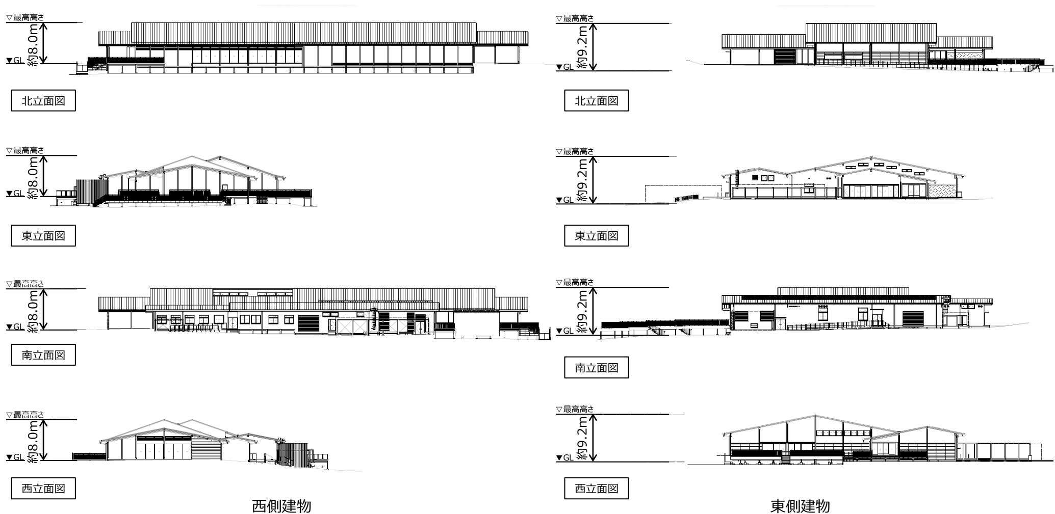
立 面 図
