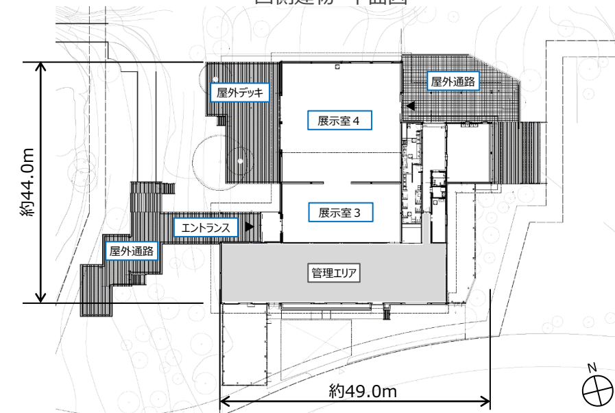
東側建物 平面図
