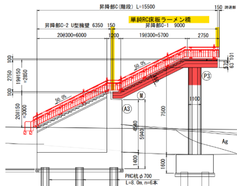
昇降部C 側面図 S=1:100
