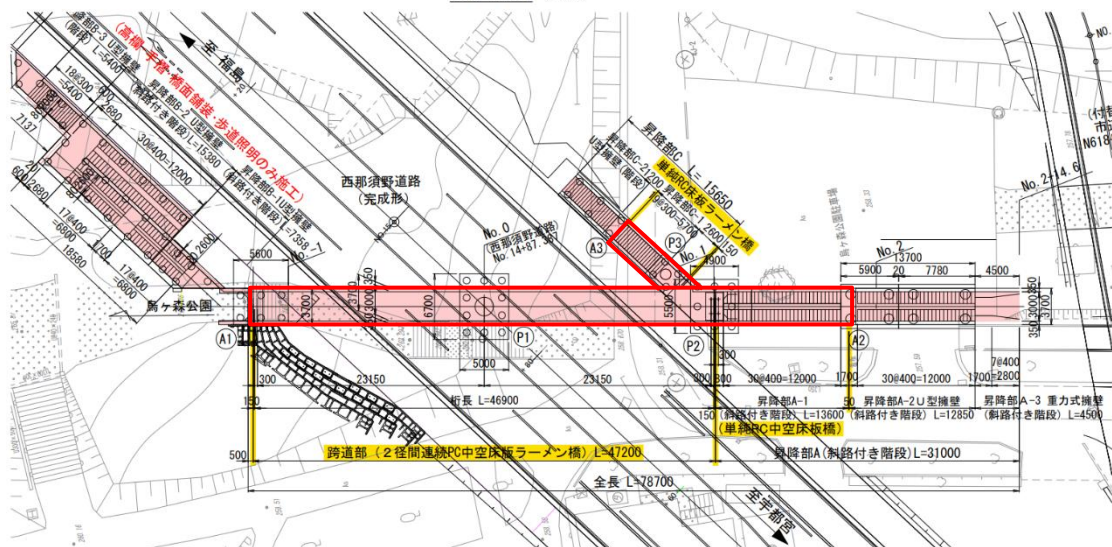
全体平面図 S=1:250
