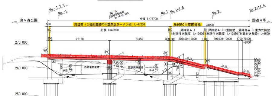
跨道部・昇降部A 側面図 S=1:250
