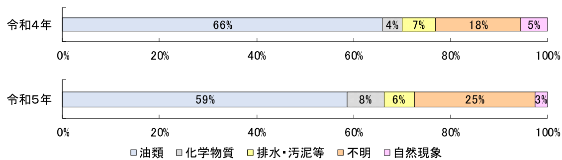
図 14 原因物質別水質事故通報件数割合
