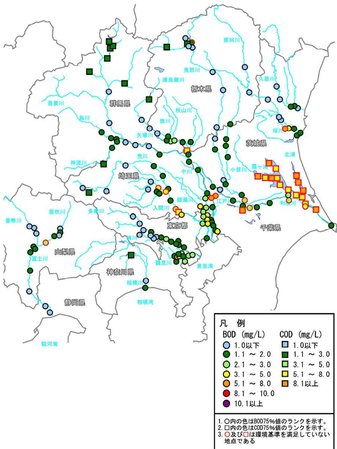
図3 令和5年 BOD・COD75%値の水質状況
