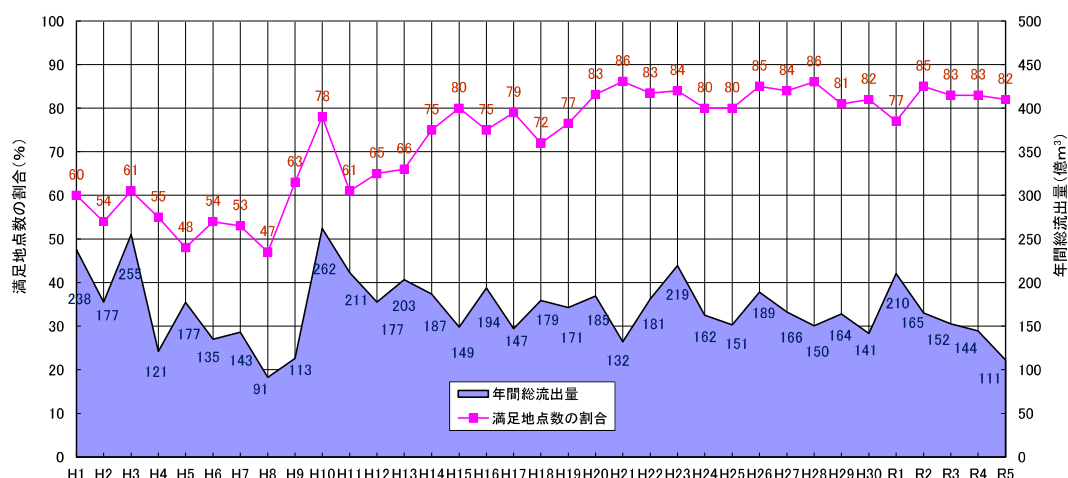
図 1 環境基準を満足している地点数の割合と河川の年間総流出量の経年変化 ※5
