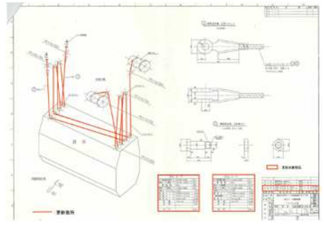
8号ゲート ワイヤロープ図
