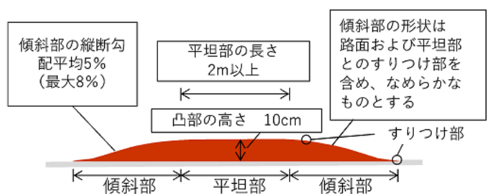
[縦断面図]
