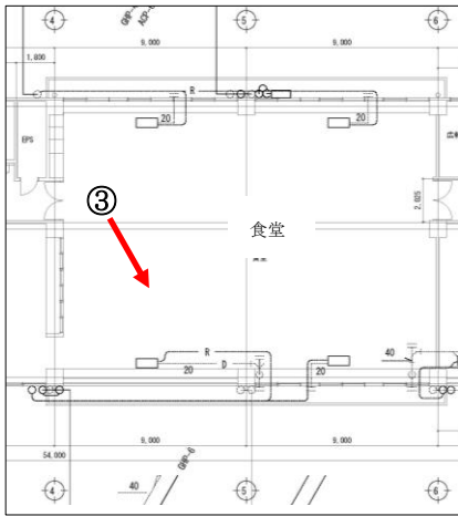
別館 2階平面図
