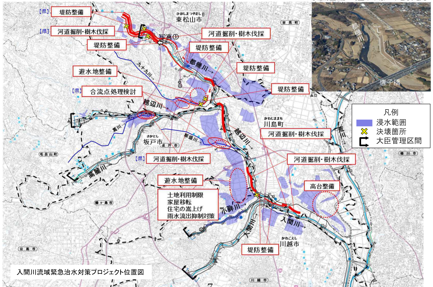
【堤防整備】埼玉県東松山市葛袋地先
