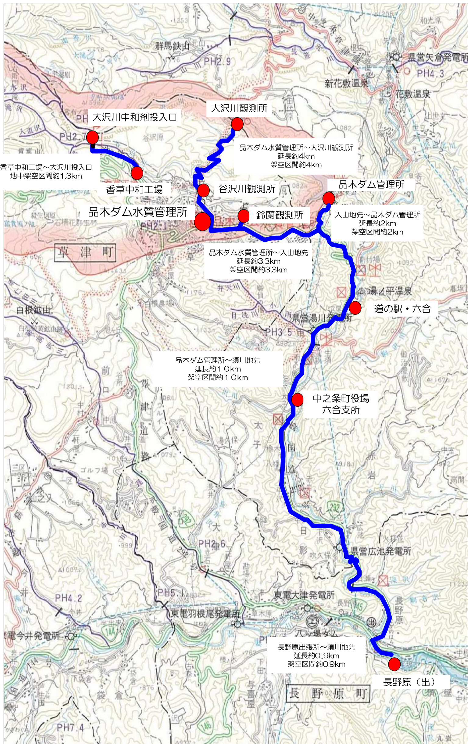
別紙一 3 品木ダム電気通信設備図
