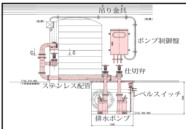
(下部監査廊) 完成イメージ図 (一部分)
