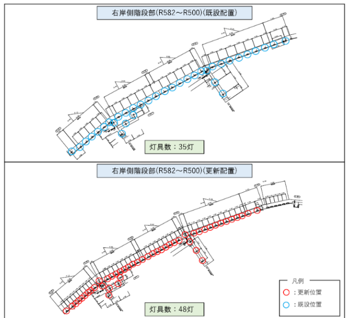
監査廊照明配置平面図（一部）
