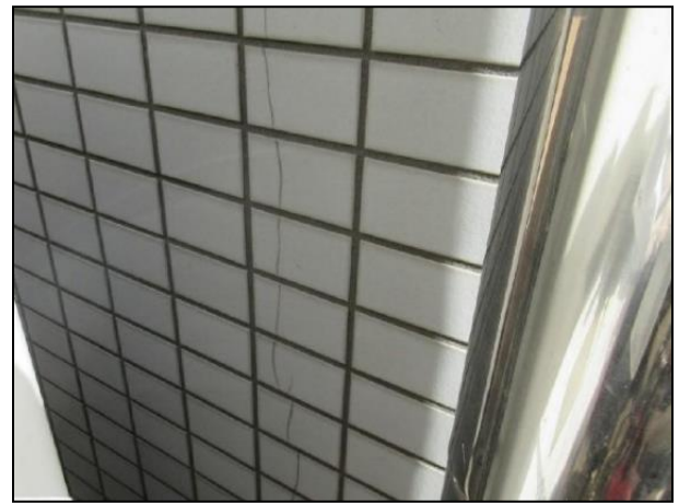
外壁タイルひび割れ状況
