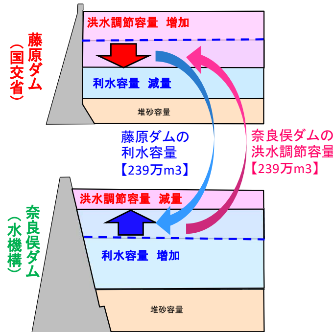
○藤原ダムおよび奈良俣ダムの貯水容量概念図
