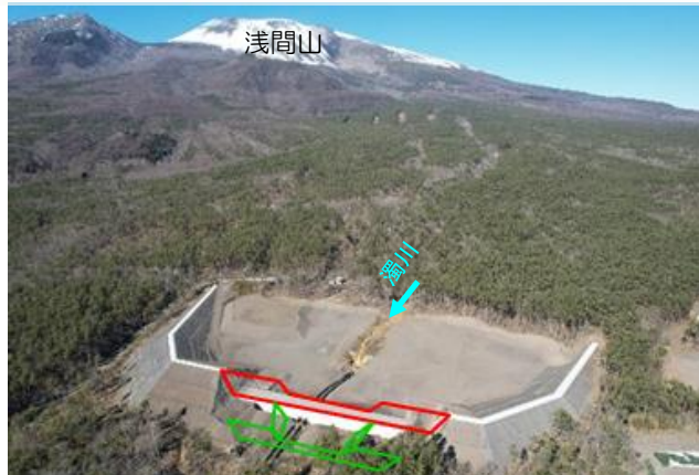
濁川第二砂防堰堤(施工中)
