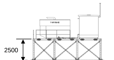
更新後発電設備
