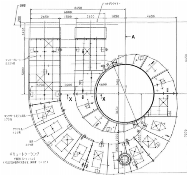
Fig.15 ダブルボリュートケーシングの平面図
