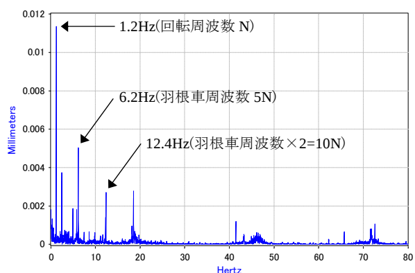
Fig.14 周波数分析結果
