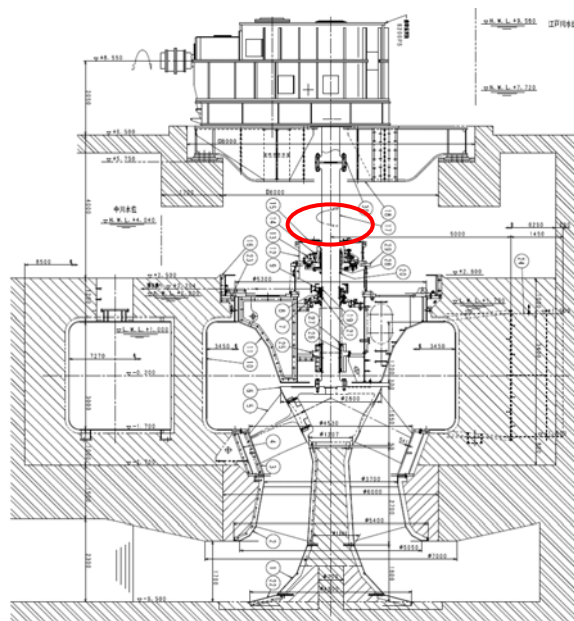
Fig.6 B排水機場のポンプ構造断面図
