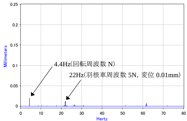
Fig.9 周波数分析結果（整備前）
