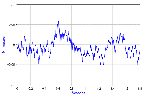
Fig.13 振動波形
