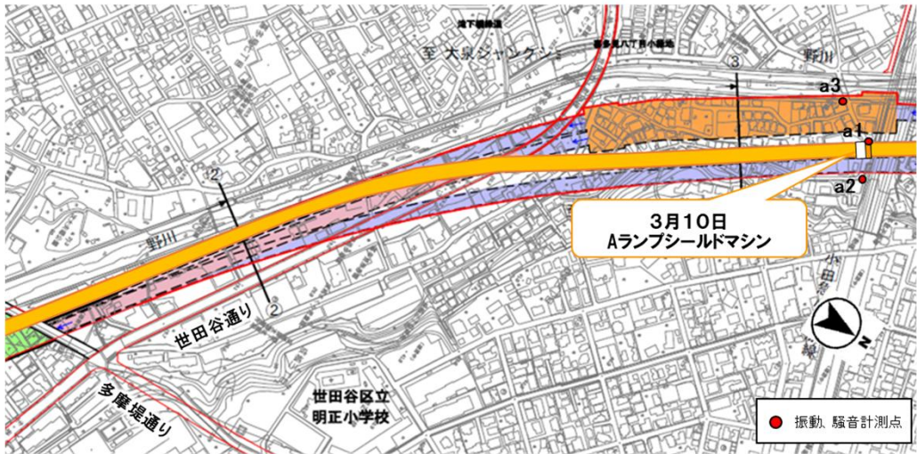
【3月10日(火)シールドマシン位置図】
