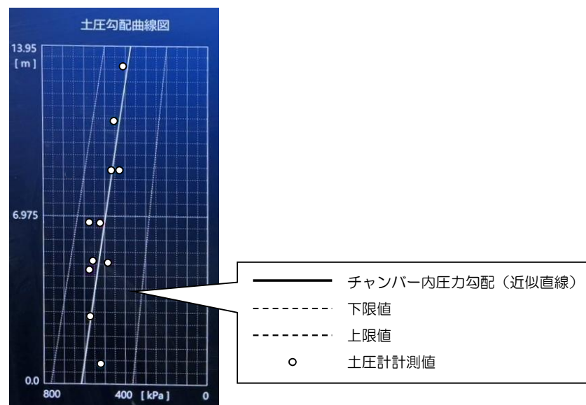
チャンバー内圧力勾配リアルタイム監視状況（762R）
