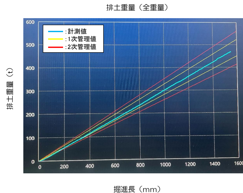
排土重量リアルタイム監視状況（689R）
