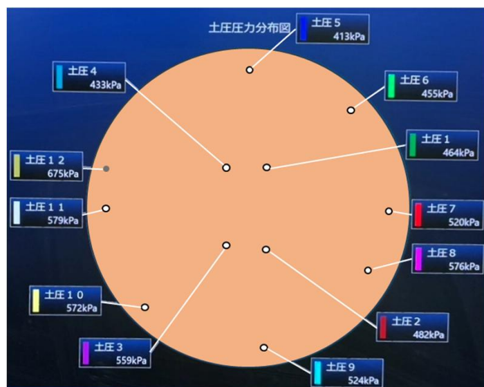
チャンバー内土圧計配置図（切羽から坑口を望む）
