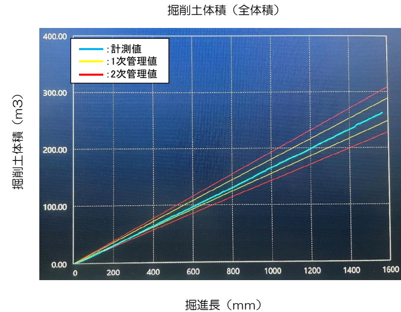
掘削土体積リアルタイム監視状況（689R）
