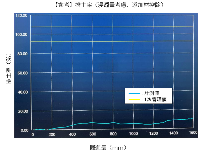
排土率リアルタイム監視状況（689R）
