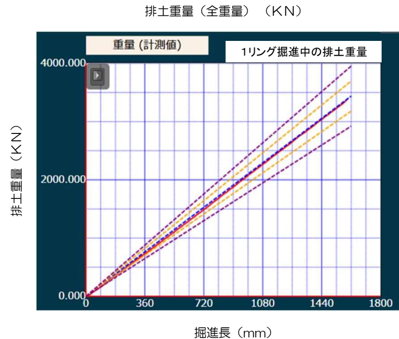
排土重量リアルタイム監視状況（186R）
