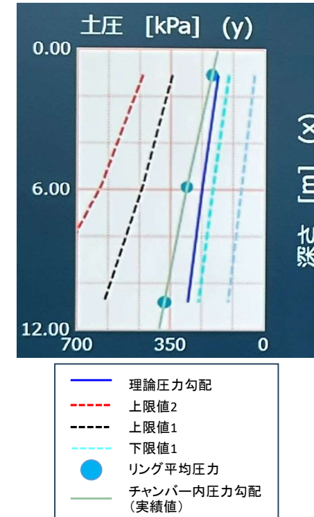
チャンバー内圧力勾配リアルタイム監視状況 (228R)
