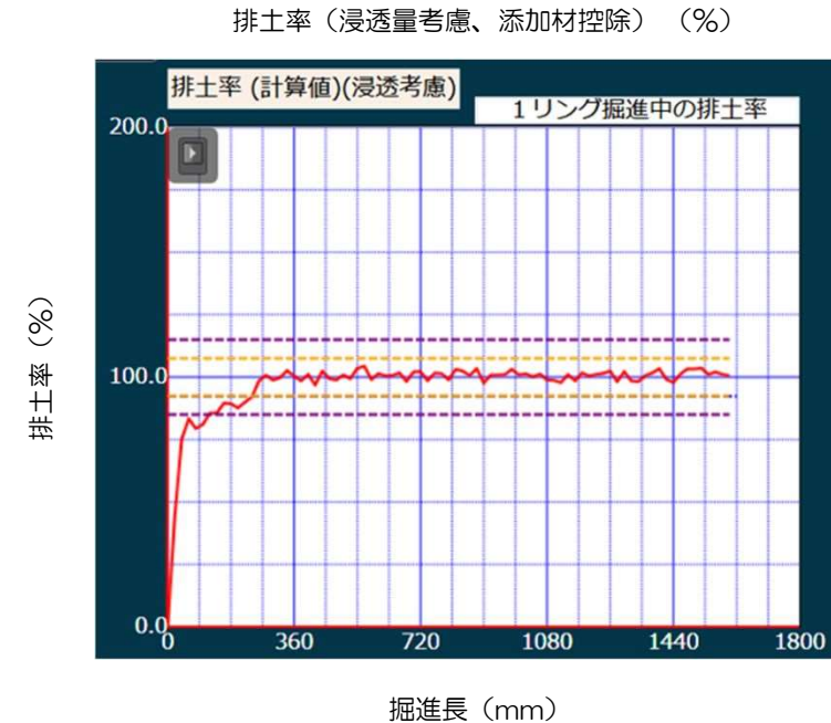
排土率リアルタイム監視状況（186R）
