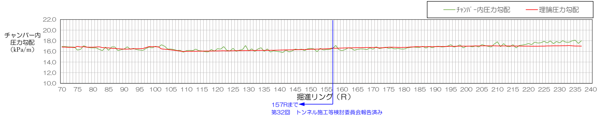
チャンバー内圧力勾配リアルタイム監視状況 (228R)
