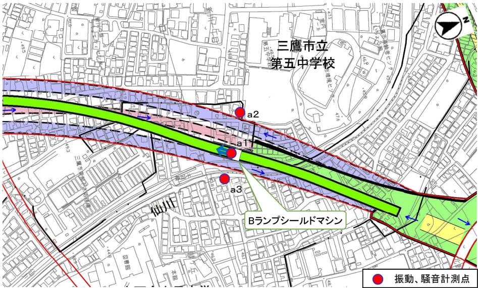
【 5月28日（水）7:30～17:00 振動・騒音計測結果（確定値）】
