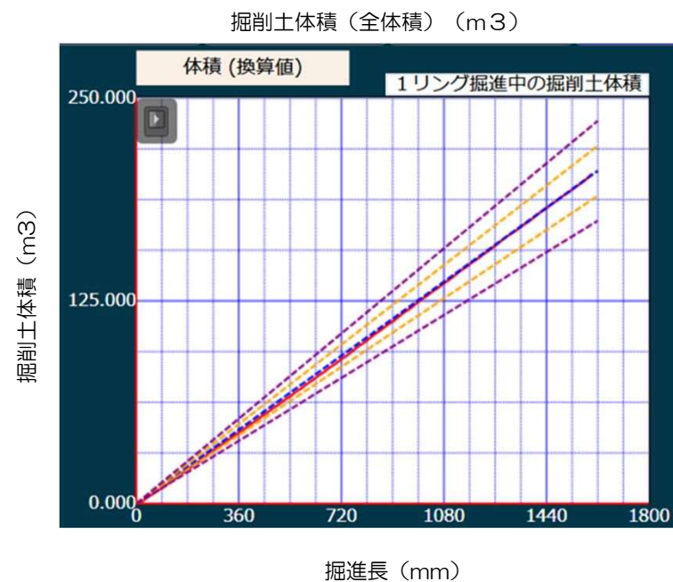
排土体積リアルタイム監視状況（186R）
