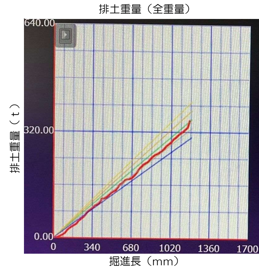
排土重量リアルタイム監視状況（623R）
