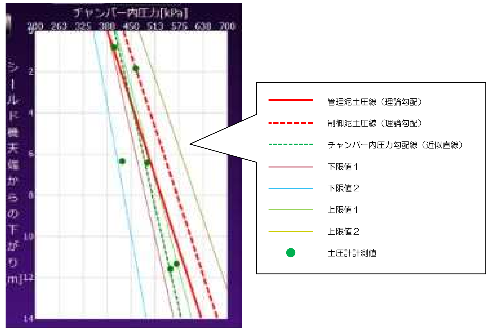
チャンバー内圧力勾配リアルタイム監視状況（623R）
