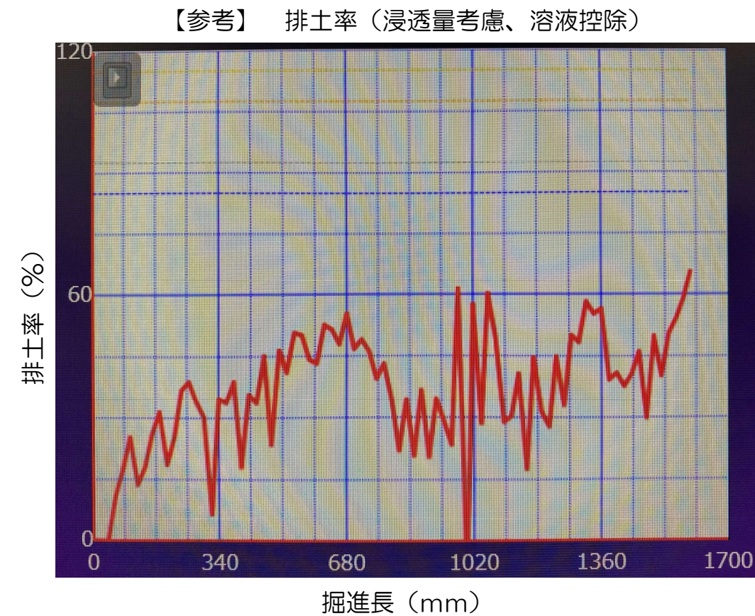
排土率リアルタイム監視状況（623R）
