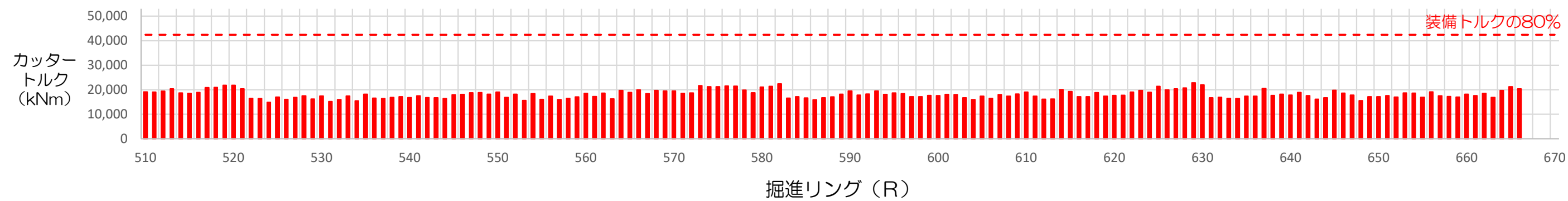
カッタートルクのリアルタイム掘進状況 (623R)
