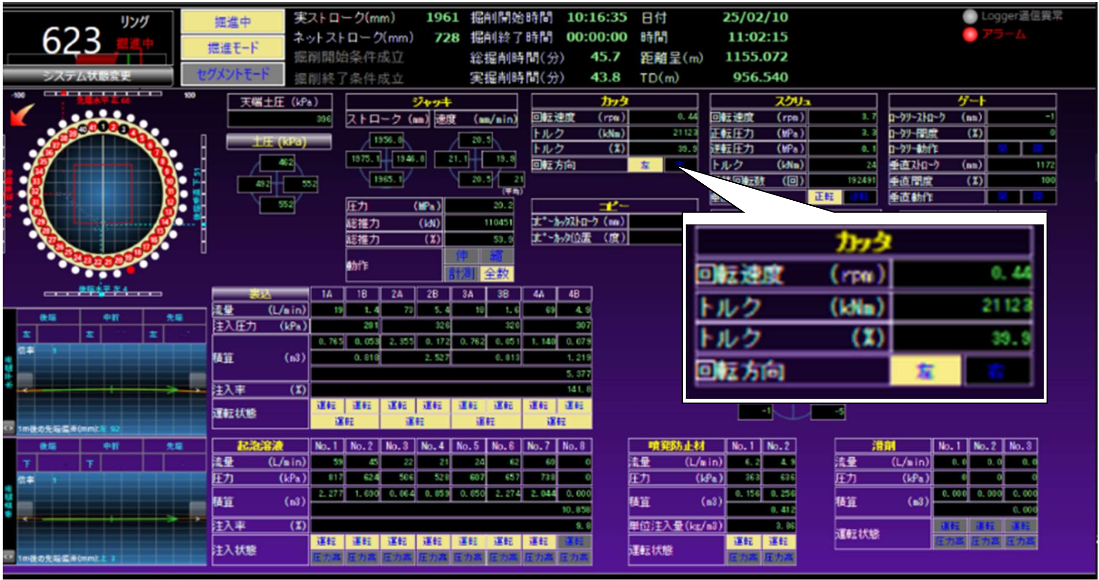
カッタートルクのリアルタイム掘進状況 (623R)
