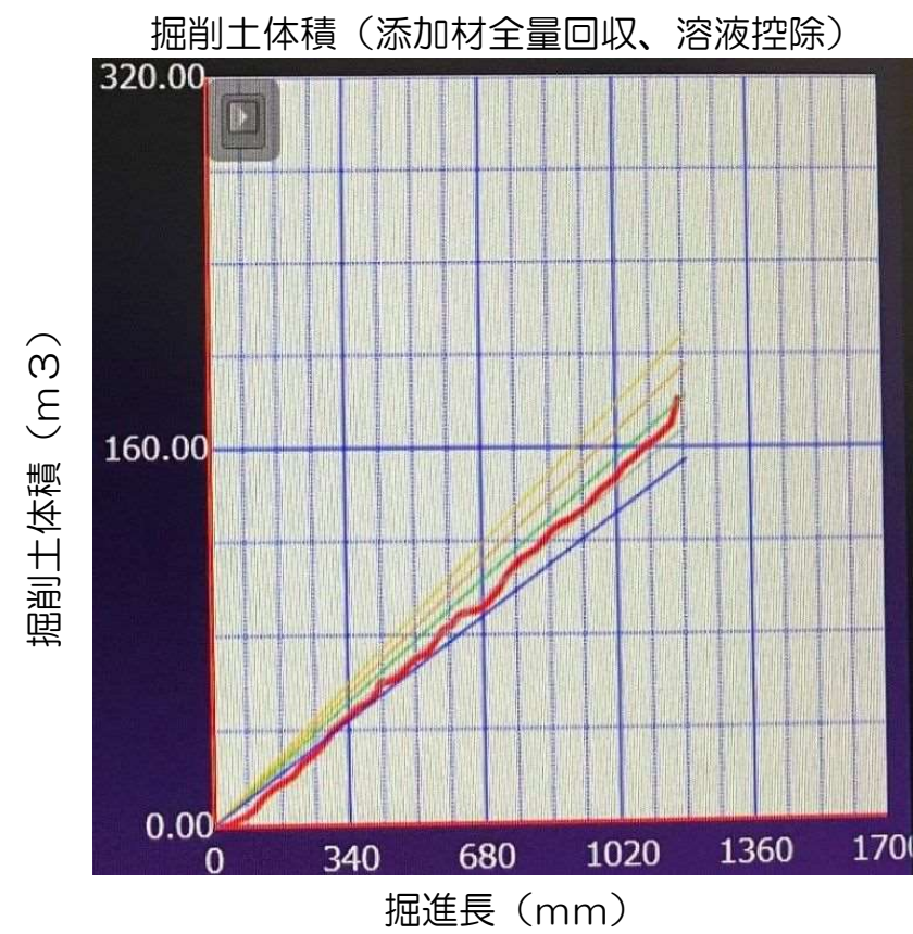
掘削土体積リアルタイム監視状況（623R）
