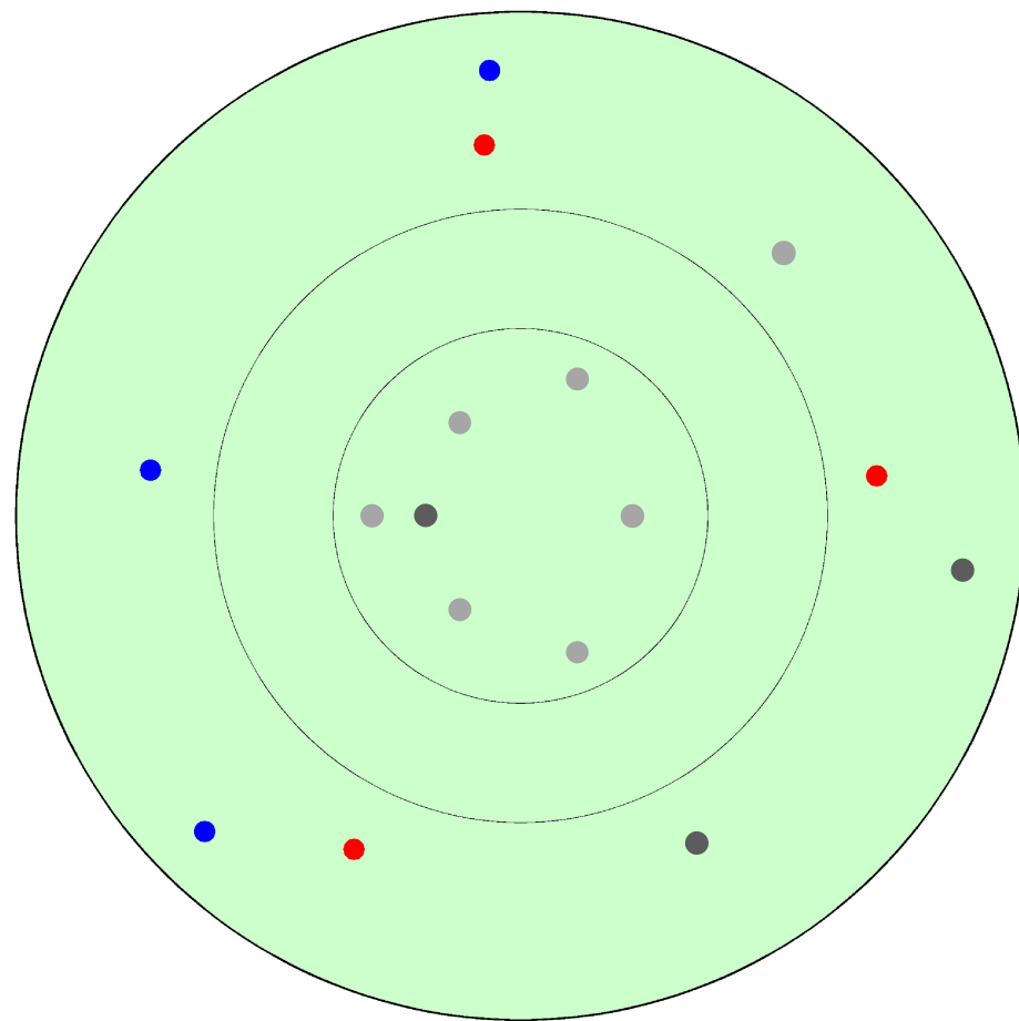
チャンバー内土圧計配置図（切羽から坑口を望む）
