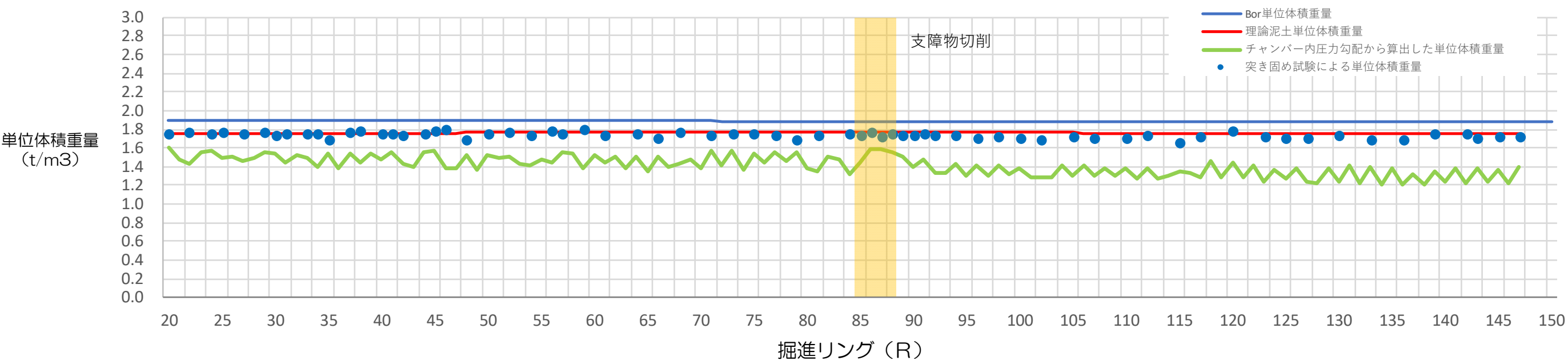
チャンバー内圧力勾配から推定した単位体積重量
