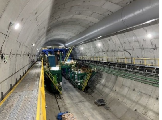
後続台車背面
