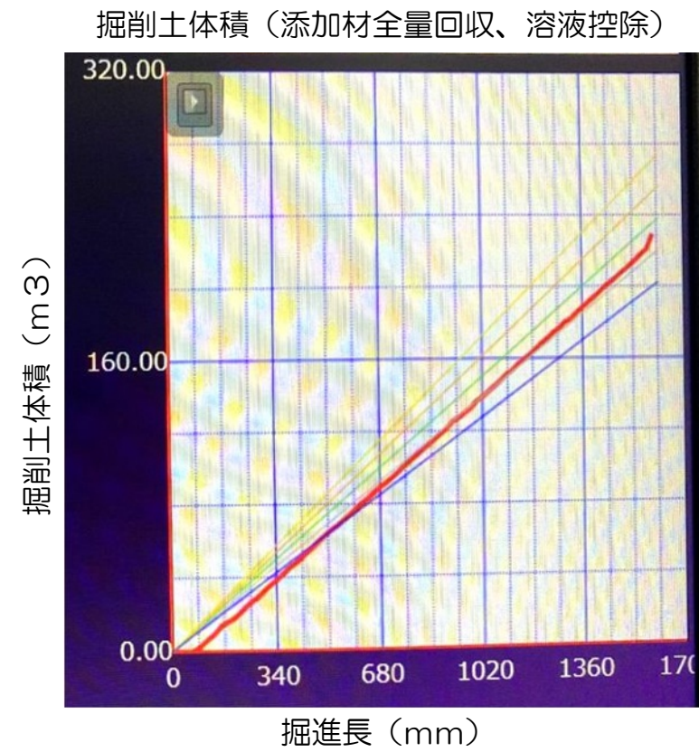
105Ring 掘削土体積リアルタイム監視状況
