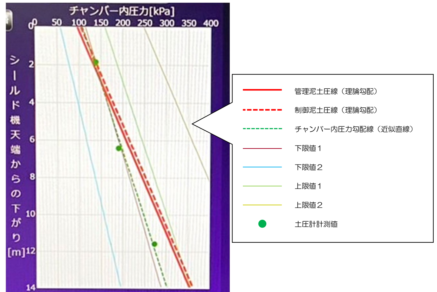
チャンバー内圧力勾配リアルタイム監視状況（105R）
