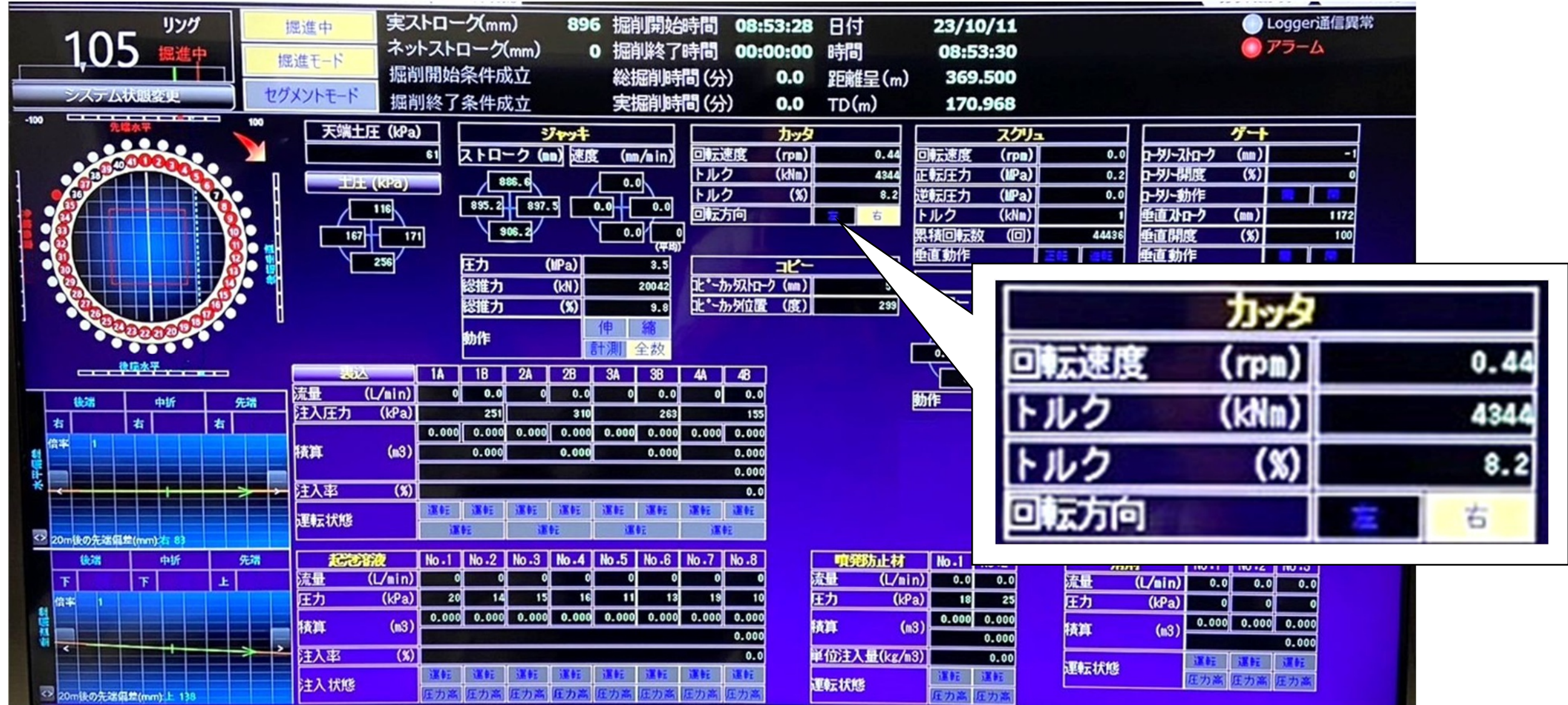
カッタートルクのリアルタイム掘進状況（105R）
