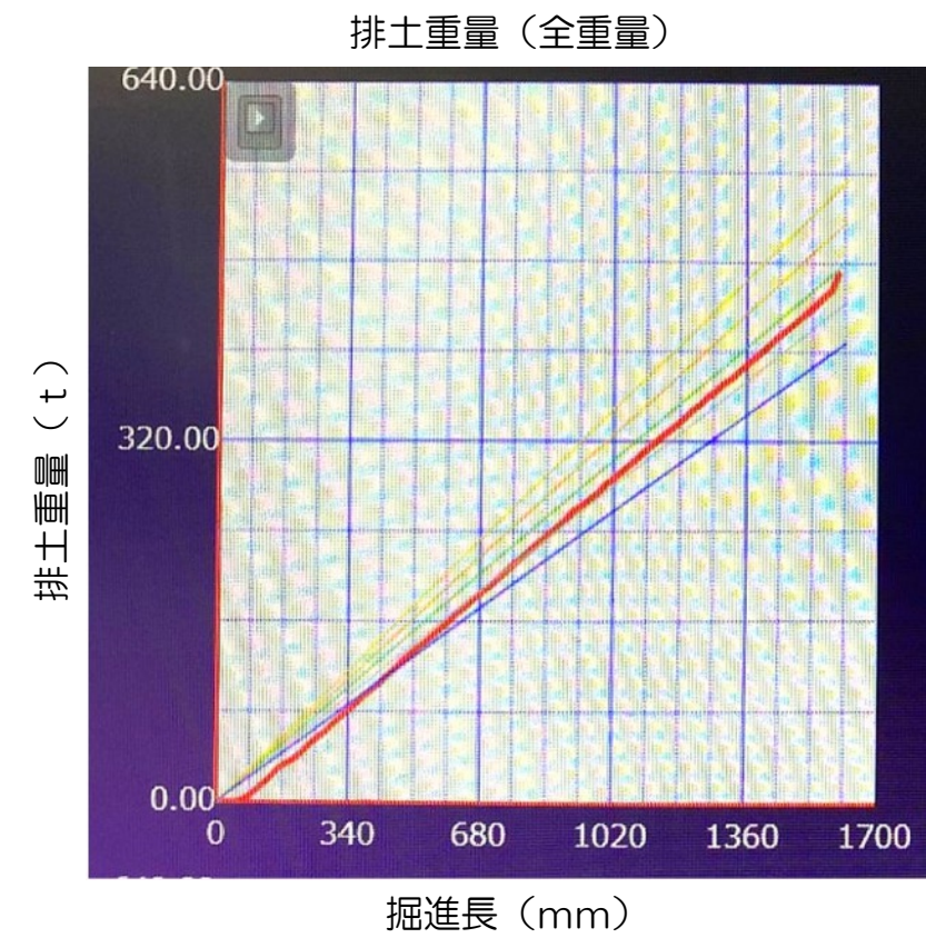
105Ring 排土重量リアルタイム監視状況
