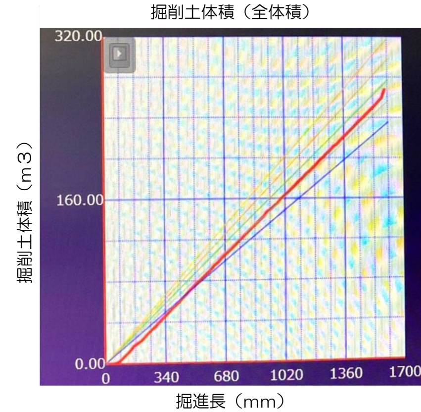
105Ring 掘削土体積リアルタイム監視状況
