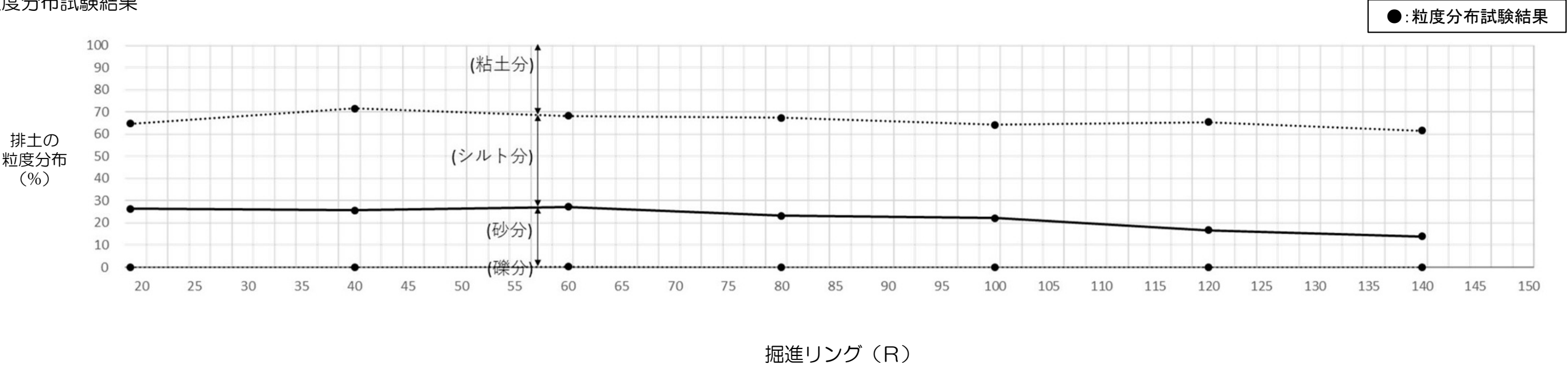
粒度分布試験結果
