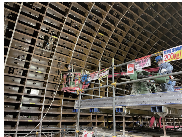
東名JCT 地中拡幅(北行) 削孔・注入
