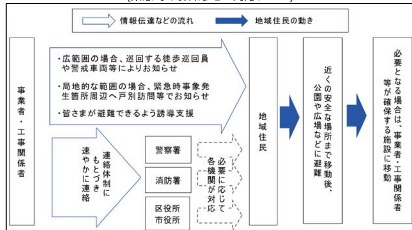
「トンネル工事の安全・安心確保の取組み」P13より抜粋
