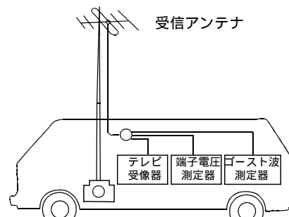
電波障害調査車両の例
