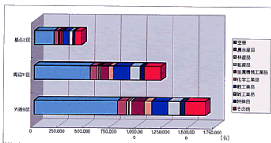
【貨物自動車の積載品目別発生・集中交通量】
