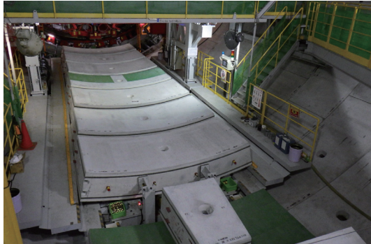
本線トンネル(南行) 立坑内セグメント供給の状況
