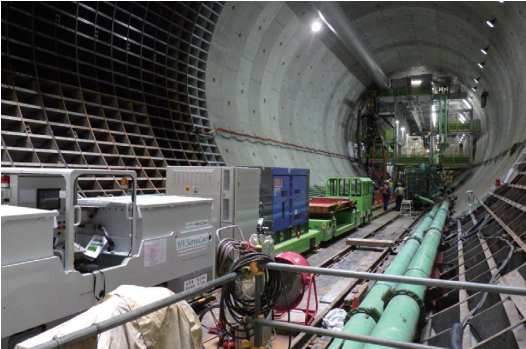
本線トンネル(南行) シールドマシン後方からの状況
