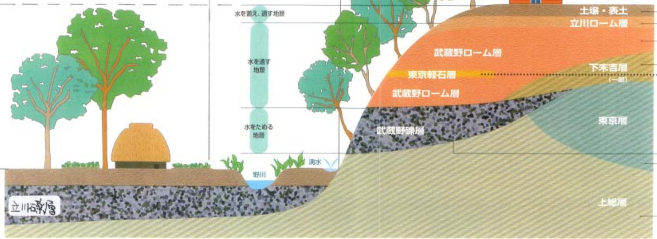
国分寺崖線の地層の成り立ち
