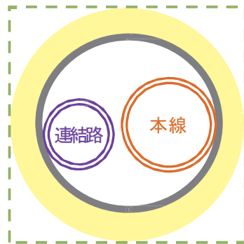
地中拡幅部のイメージ (断面図)
