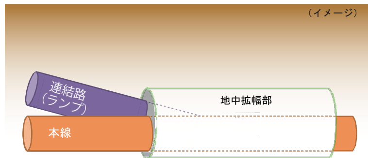
地中拡幅部のイメージ (縦断面図)
