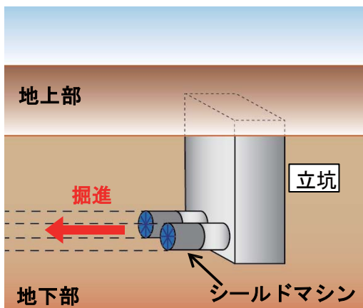
立坑及びシールド掘進のイメージ
