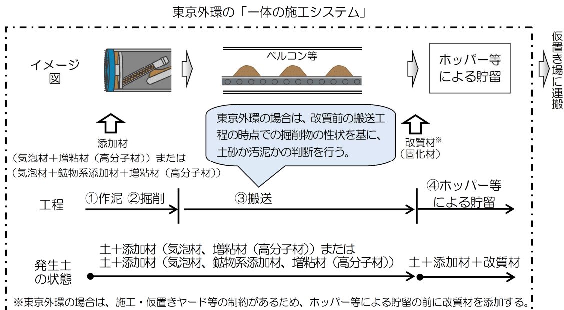
図-2.3 東京外環の「一体の施工システム」
