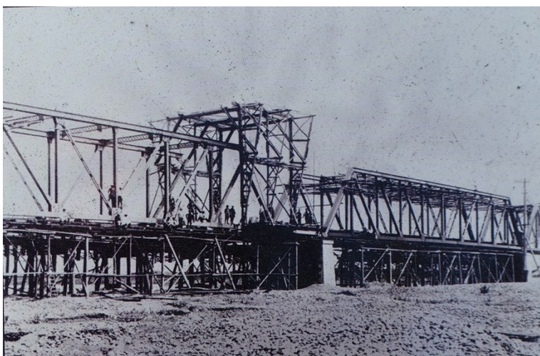
1922（大正11）年～1924（大正13）年 九連トラス橋の工事
