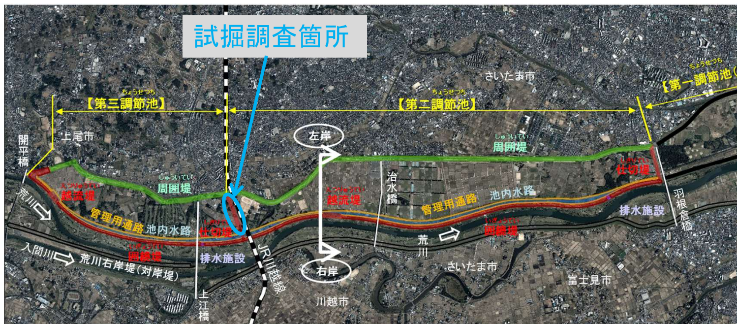
計画平面図
