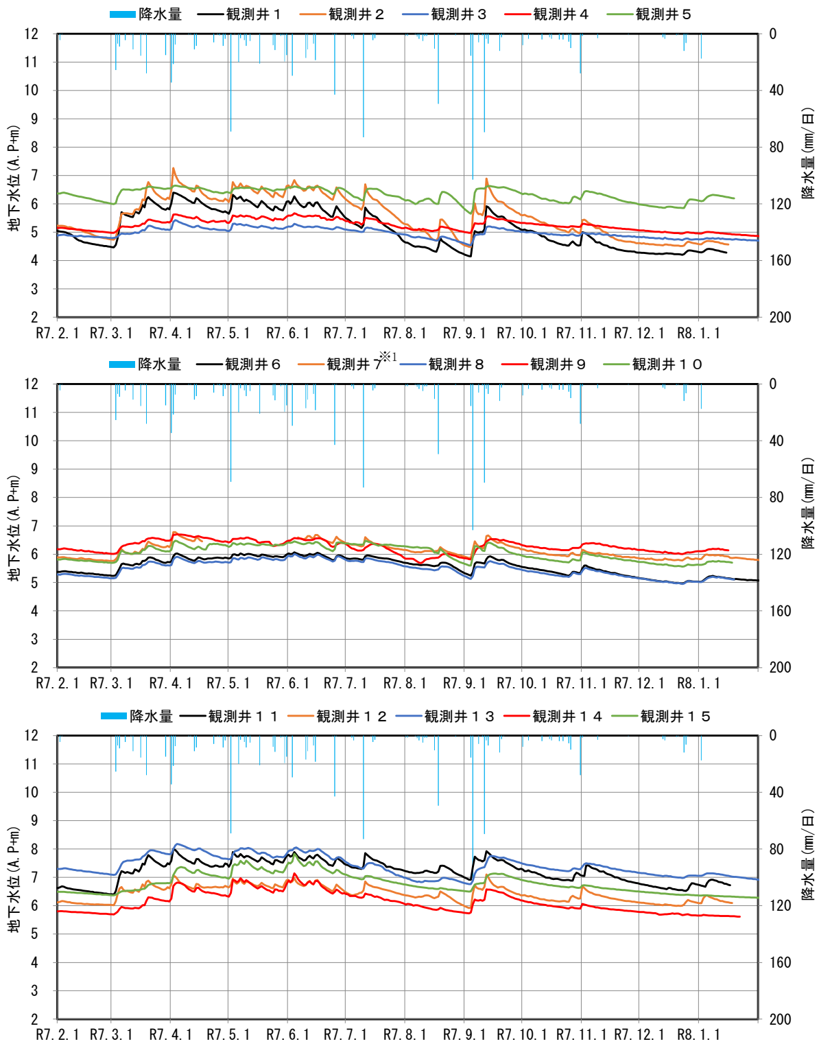
図 6 地下水位のモニタリング結果（令和7年2月～令和8年1月）
