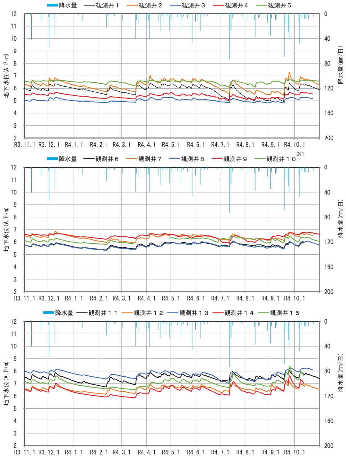
図4 地下水位のモニタリング結果（令和3年11月～令和4年10月）
