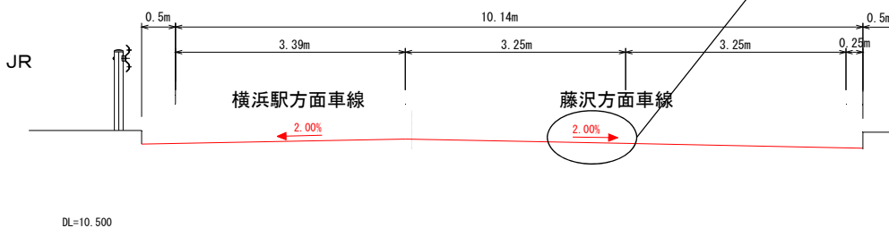
横断面図（対策後）A-A断面
