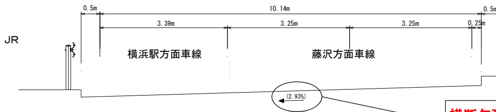
横断面図（対策後）A-A断面
