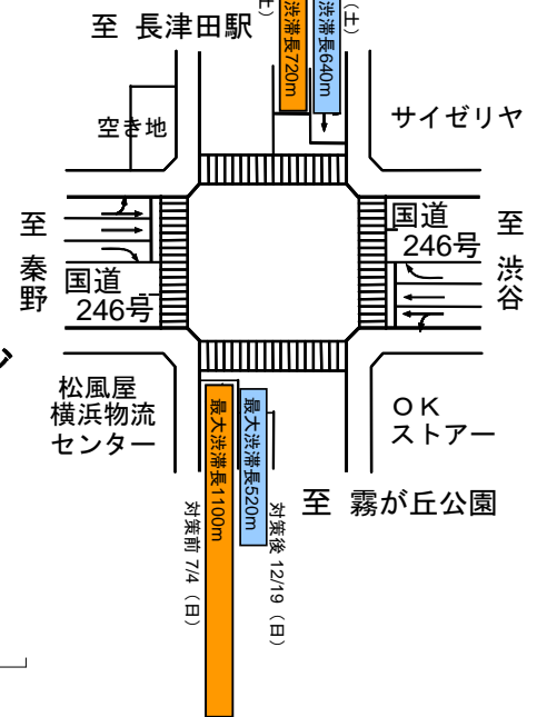
交差点平面図 (最大渋滞長の変化)
