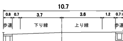
標準横断面図（現況）
