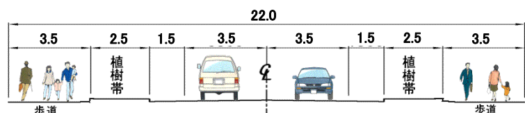
標準横断面図（計画）
